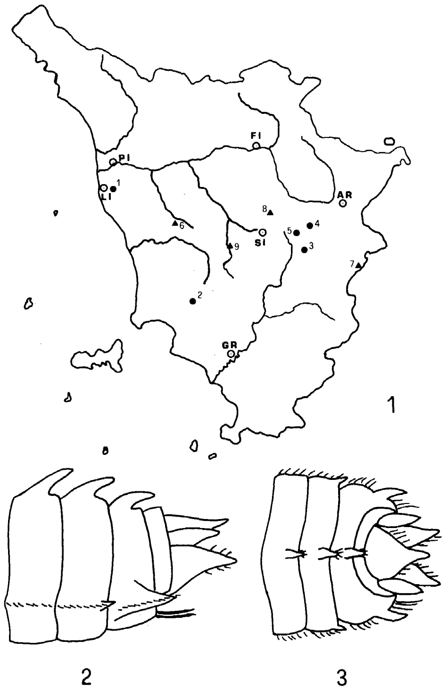
Fig. 1: cartina della Toscana con la sigla di alcune città capoluogo di provincia (FI: Firenze; PI: Pisa; LI: Livorno; AR: Arezzo; SI: Siena; GR: Grosseto). I dischi neri indicano le stazioni note in bibliografia di Somatochlora meridionalis Nielsen, 1935; i triangoli stanno invece ad indicare le stazioni inedite, riportate dall'A. nella presente nota. Elenco delle stazioni: 1) Livorno; 2) lago dell'Accesa; 3) travaso della diga del Calcione; 4) t. Esse; 5) t. Lusignana; 6) Pieve di Villamagna; 7) Terontola; 8) Castellina in Chianti; 9) t. Elsa a q 185 m; fig. 2: ultimi uriti (VII-VIII-IX-X) e piramide caudale di larva di Somatochlora meridionalis Nielsen, 1935 in visione laterale; fig. 3: gli stessi in visione dorsale.
